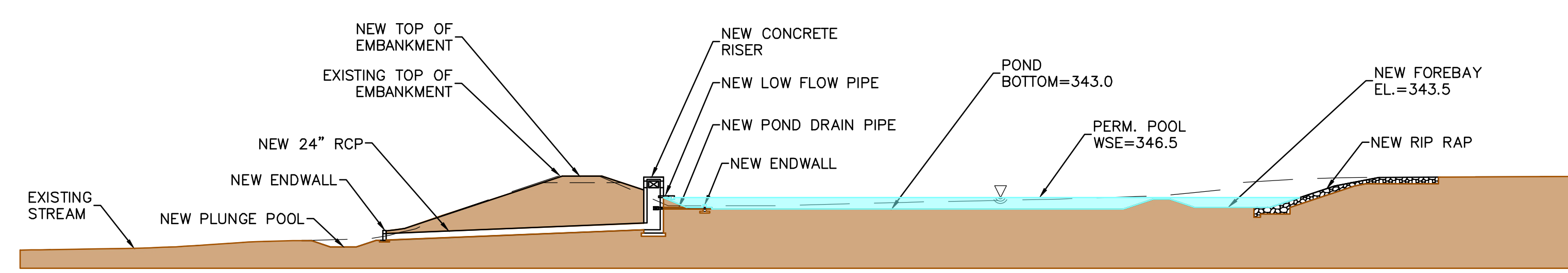
PROFILE A-A
