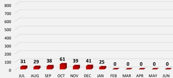
FY21- Traffic/Civil
