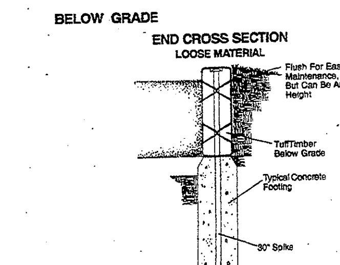
9 TOT LOT EDGING L-II SECTION 101-05 NTS
