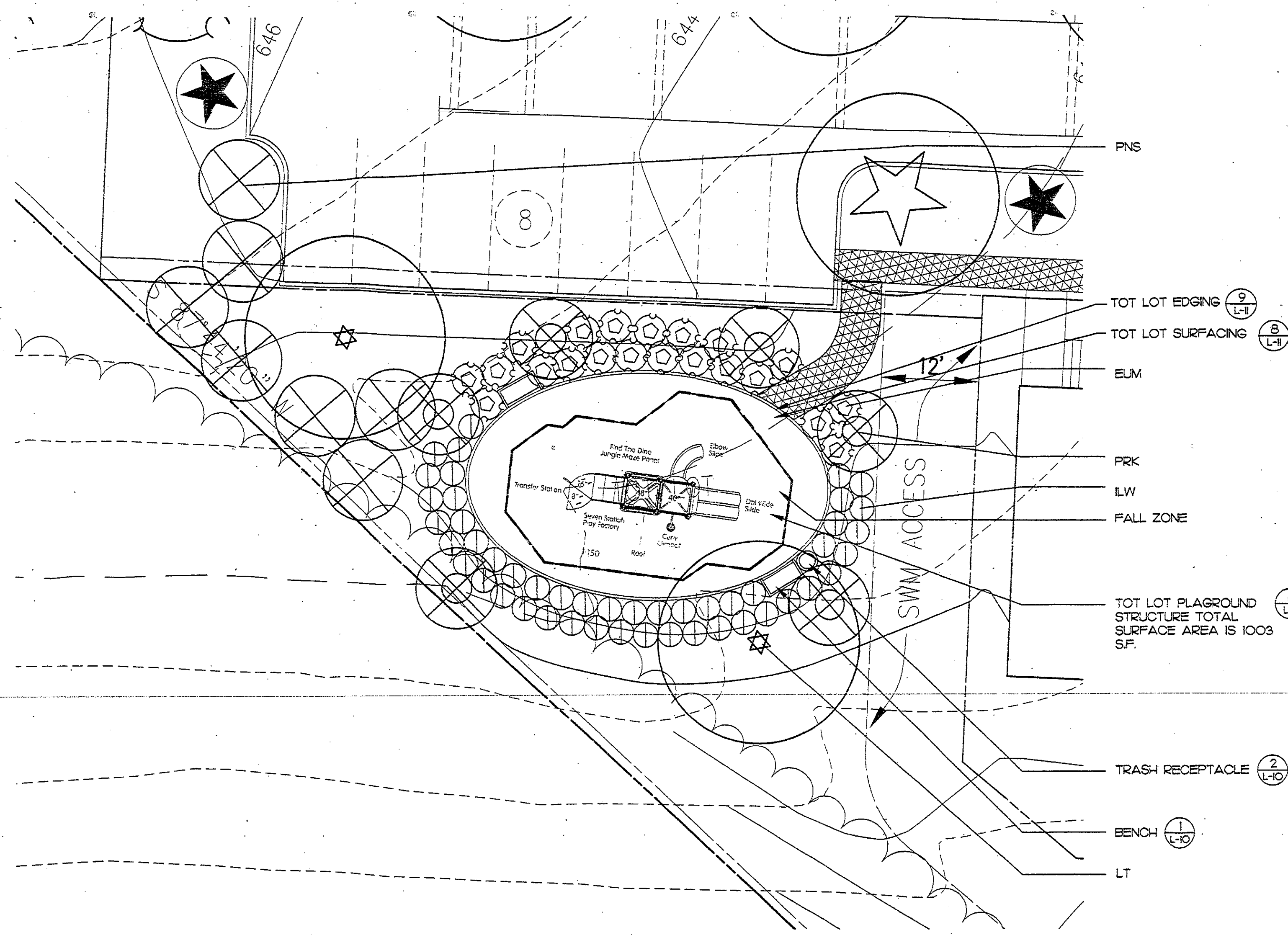
3 TOT LOT B ENLARGEMENT L-6 PLAN 1" = 10'
