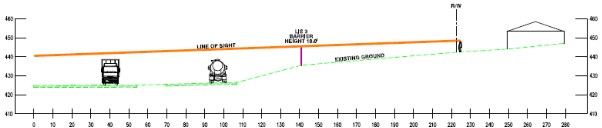
SECTION D-D
