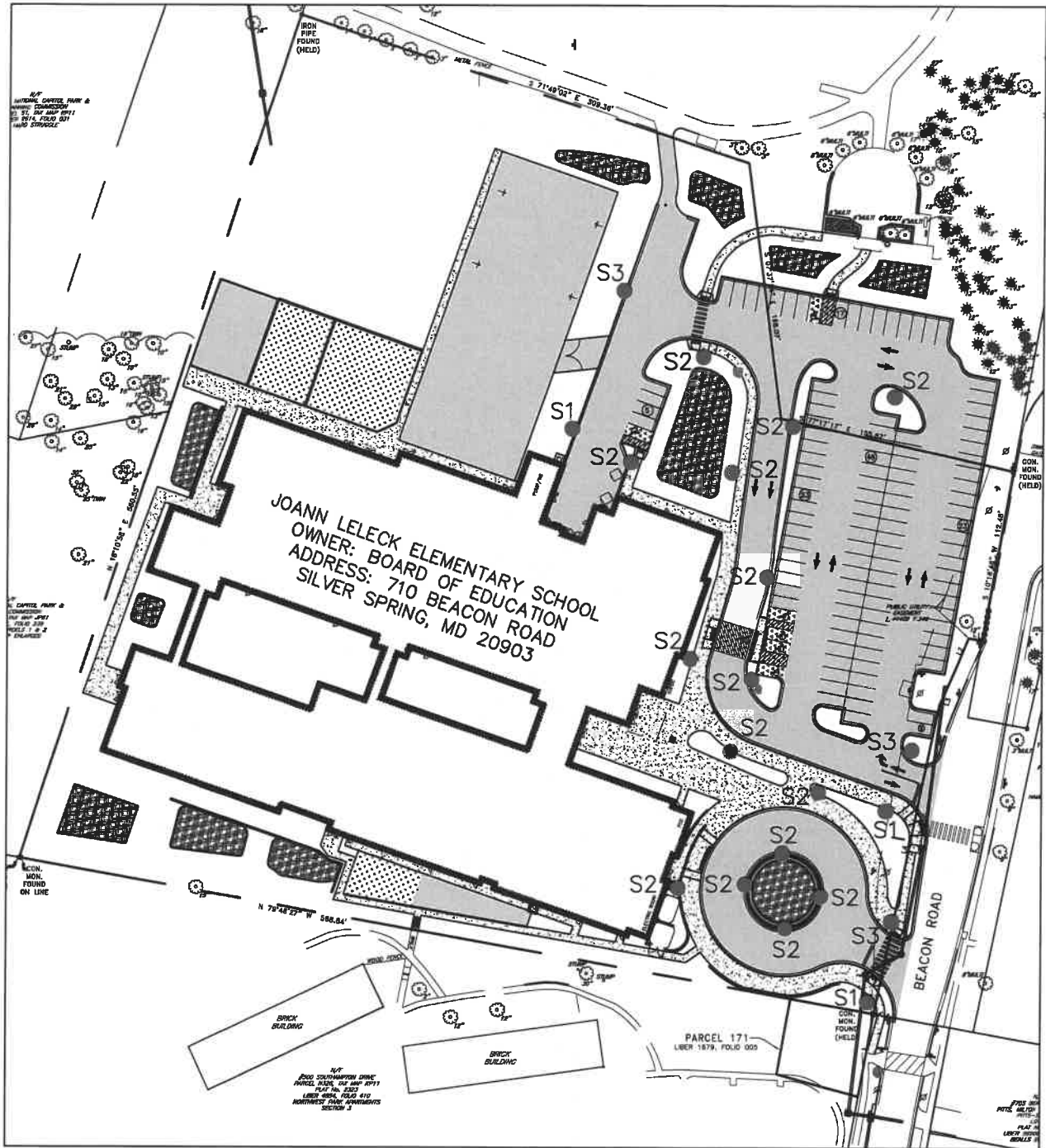
FIRE LANE PLAN SCALE: 1" = 100'
